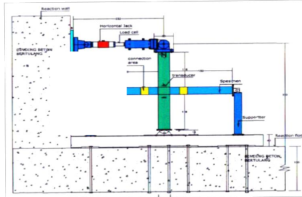
Gambar 5 Model Pengujian
